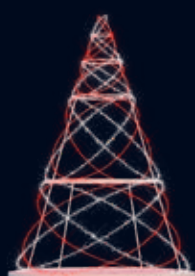
ELLIPSE XL 203845-24V H 5,85 x W 4 x D 4 x Ø 4 m 224 KG - 182 W
